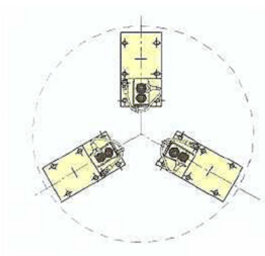
Système à 3 points d'appui
